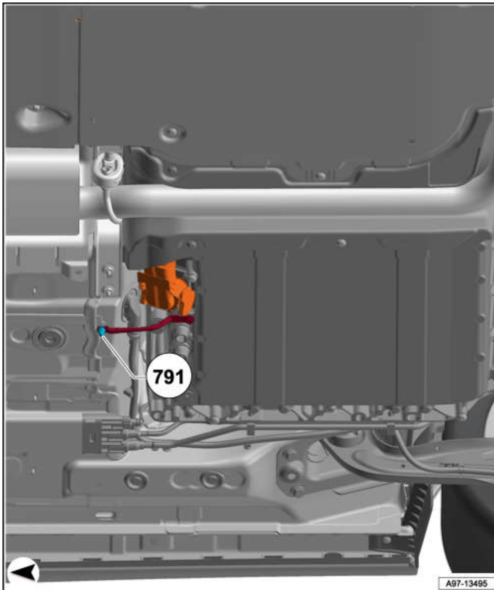
791 右 上的接地点
