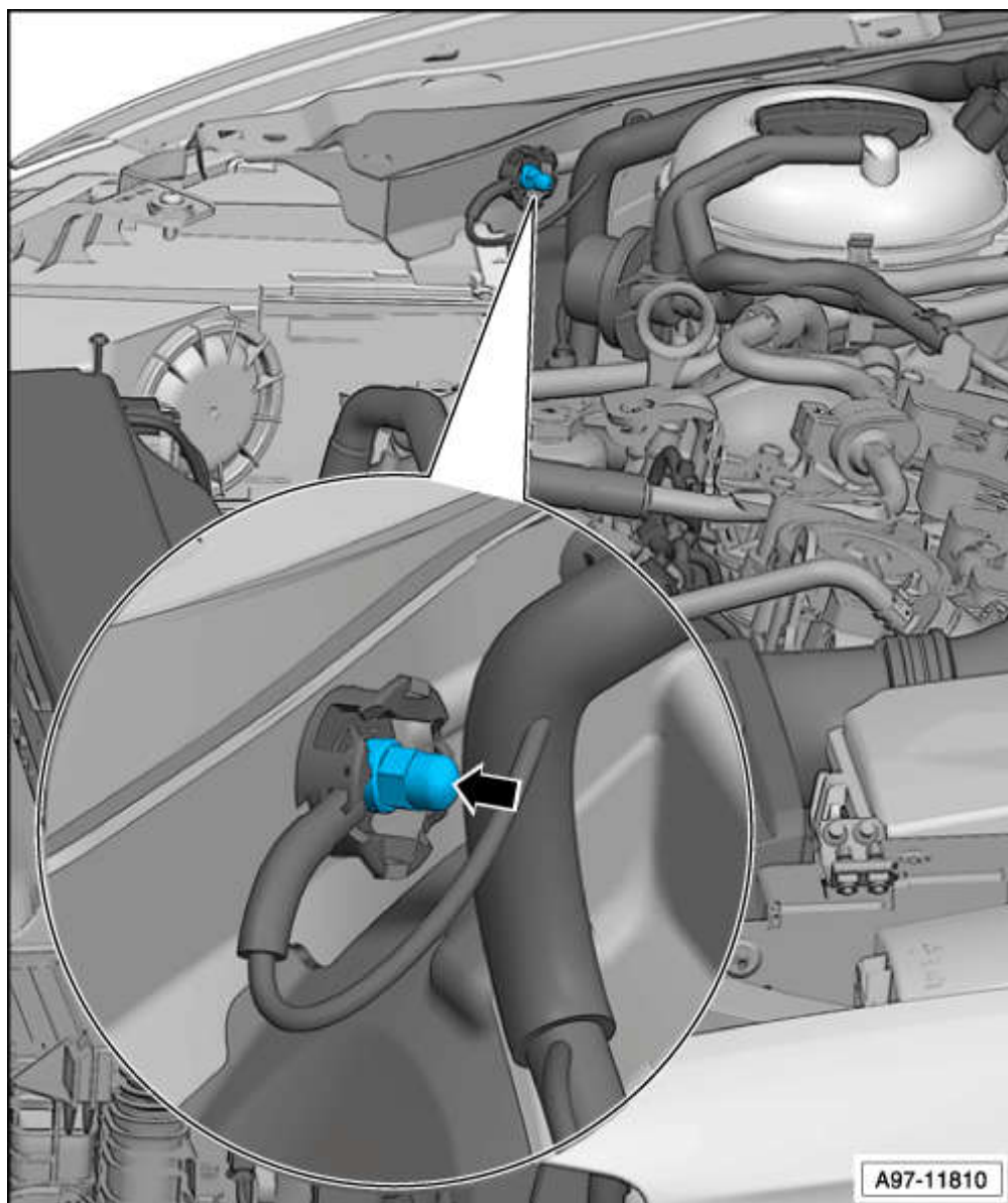
656 右大灯上的接地点 -箭头所示- 拧紧力矩 9 Nm
