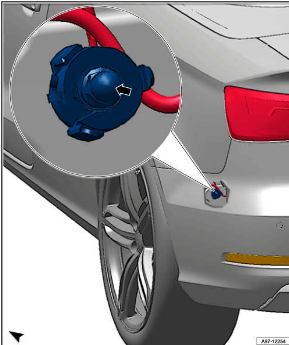
729 左 上的接地点-箭头- 拧紧力矩 9 Nm
