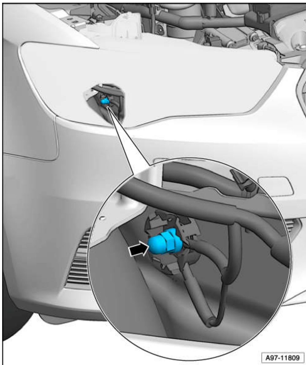
685 接地点 1 纵梁前右 -箭头- 拧紧力矩 9 Nm
